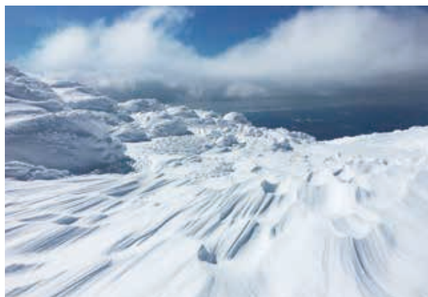
刈田岳サスツルギ
